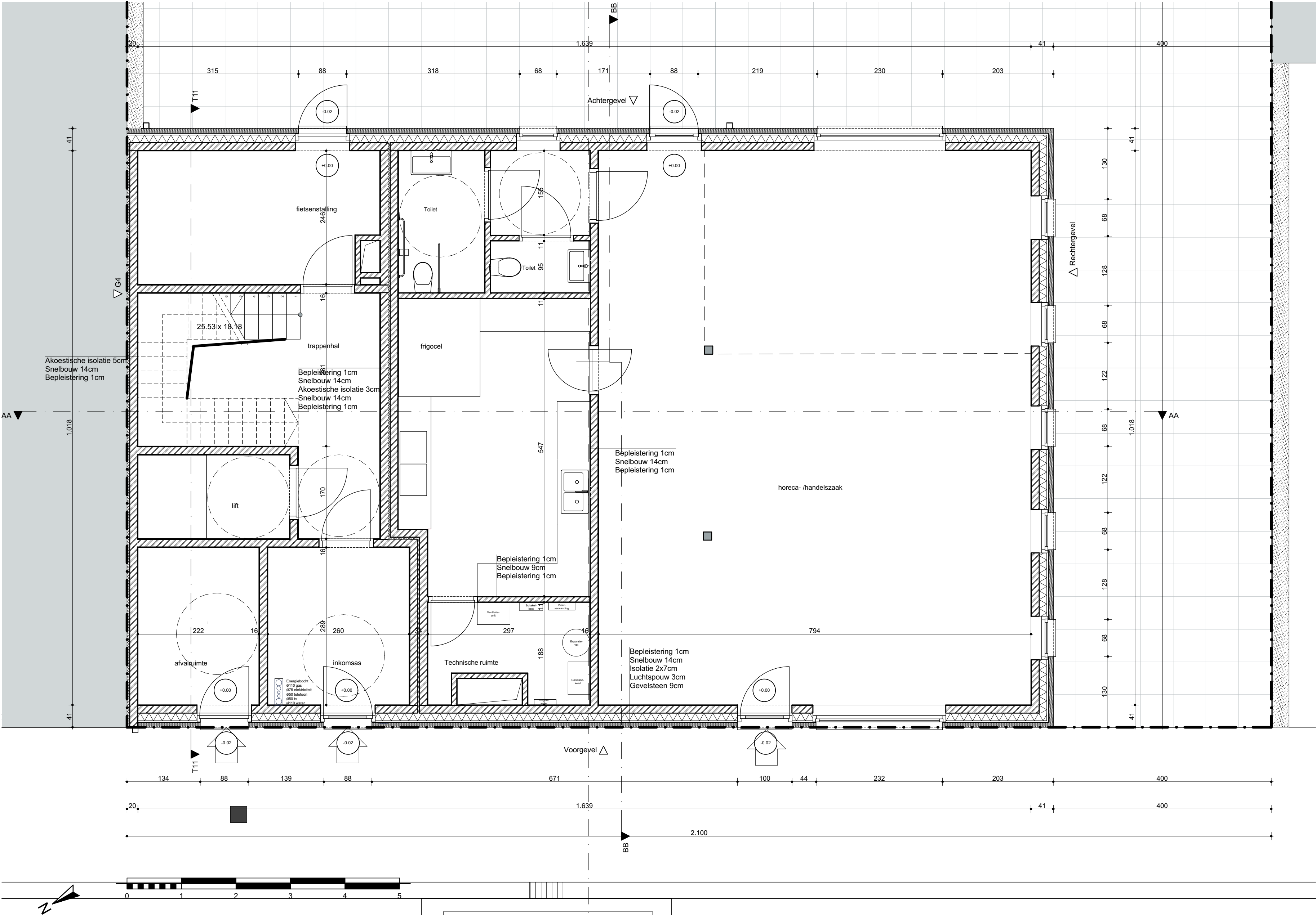
grondplan schaal 1/50
