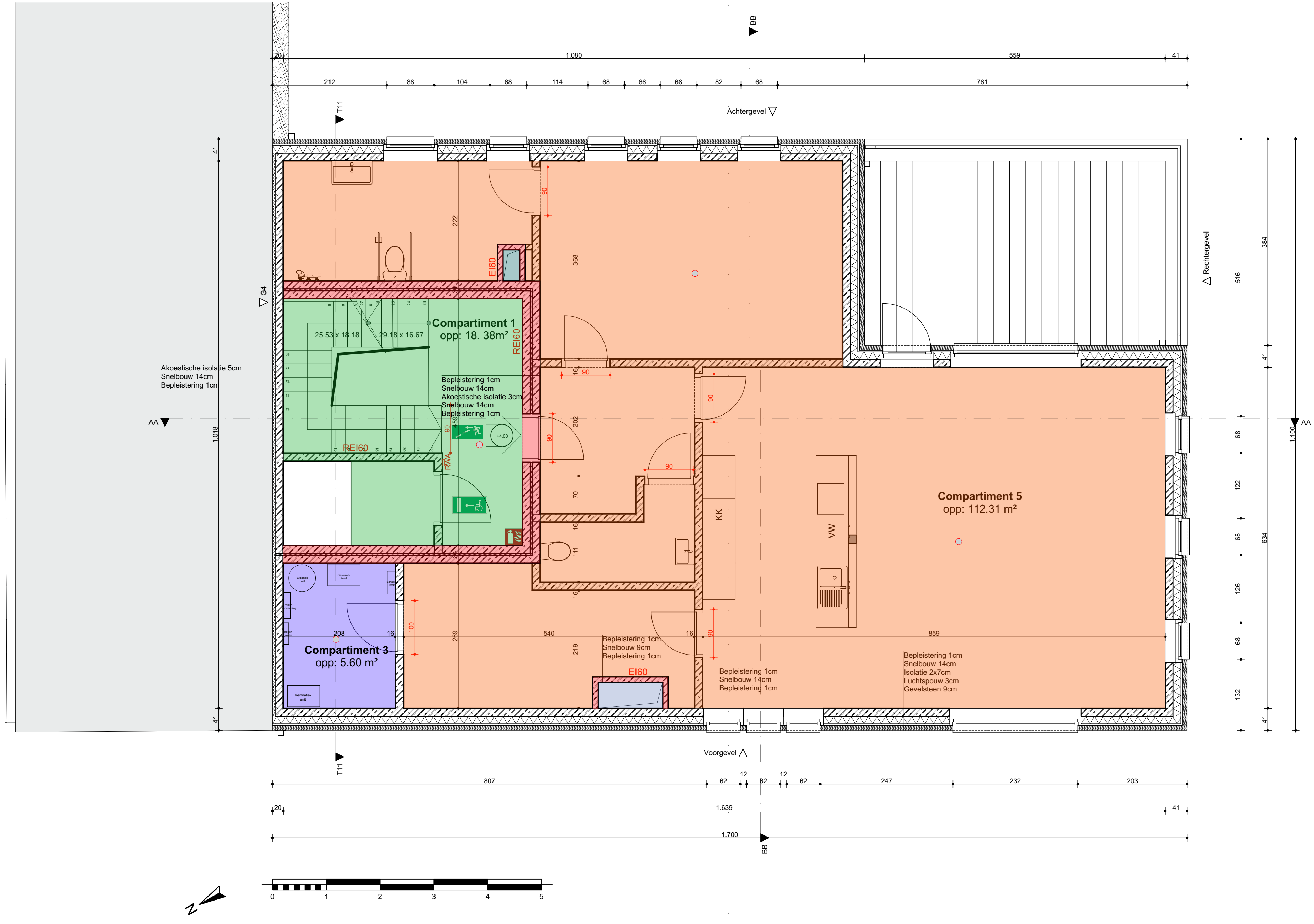
eerste verdiep brandweer schaal 1/50
