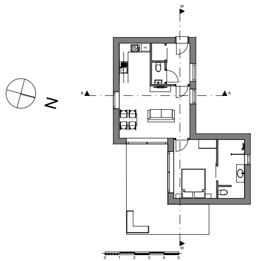
grondplan
