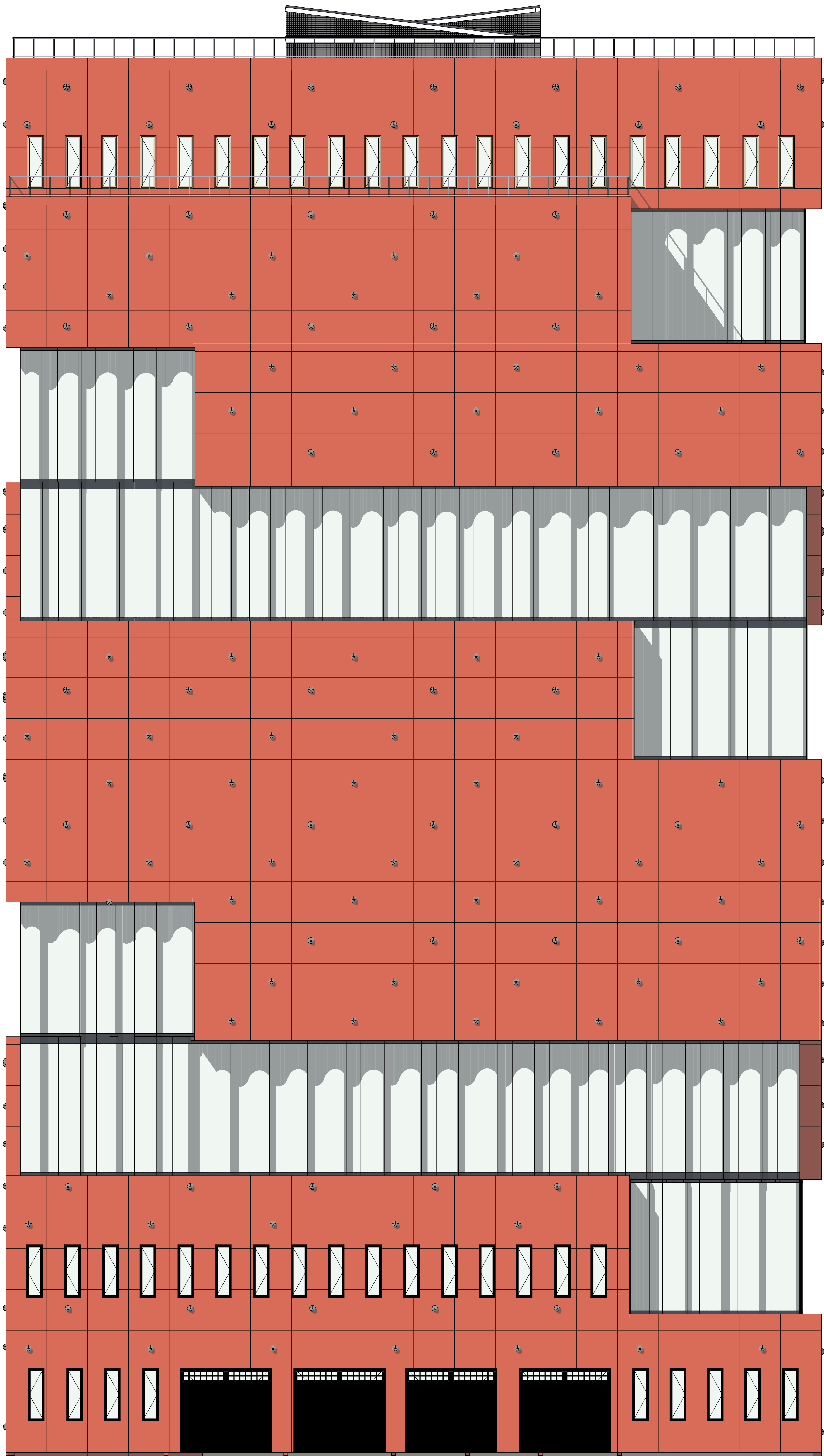
G4 Linkergevel 1:100
