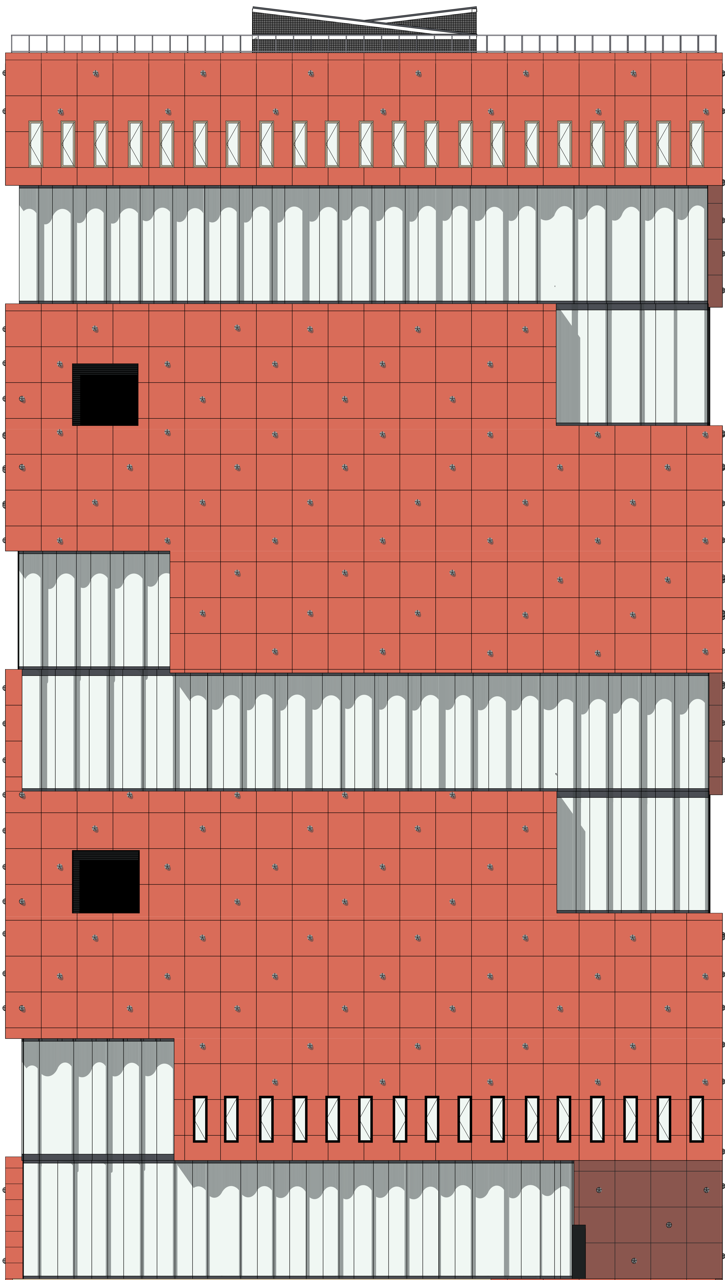
G2 Rechtergevel 1:100
