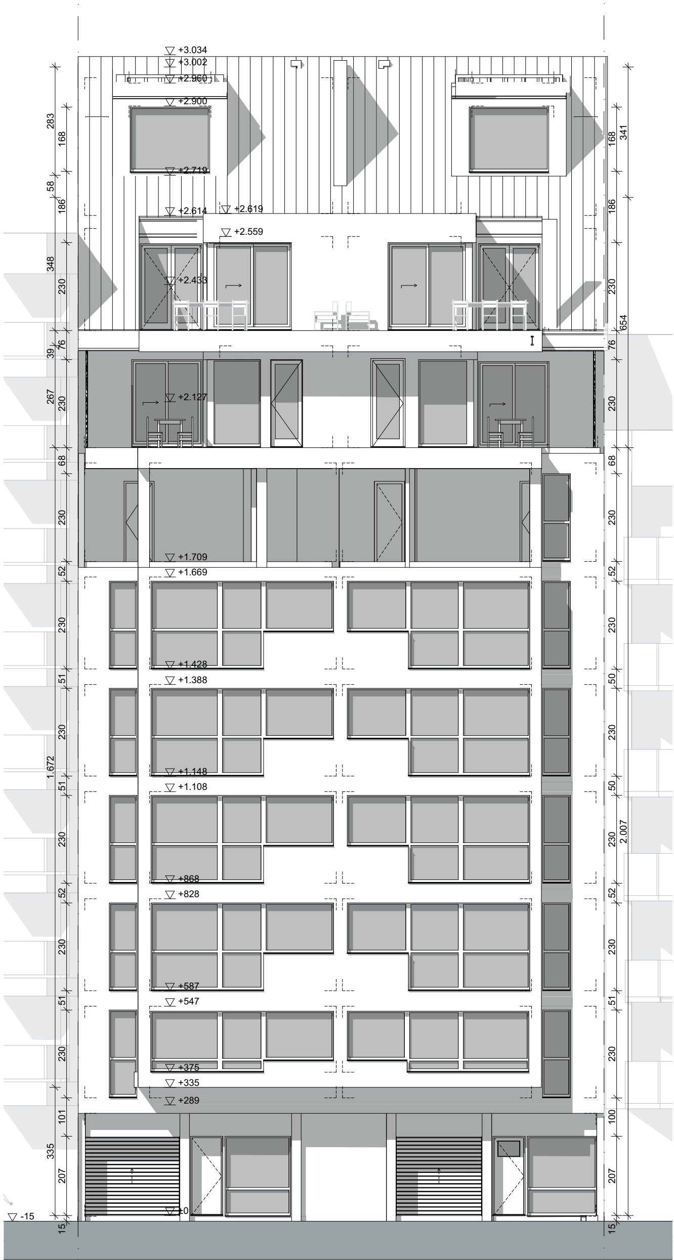
G3 Achtergevel (Jozef Dhoorelaan) 1:100
