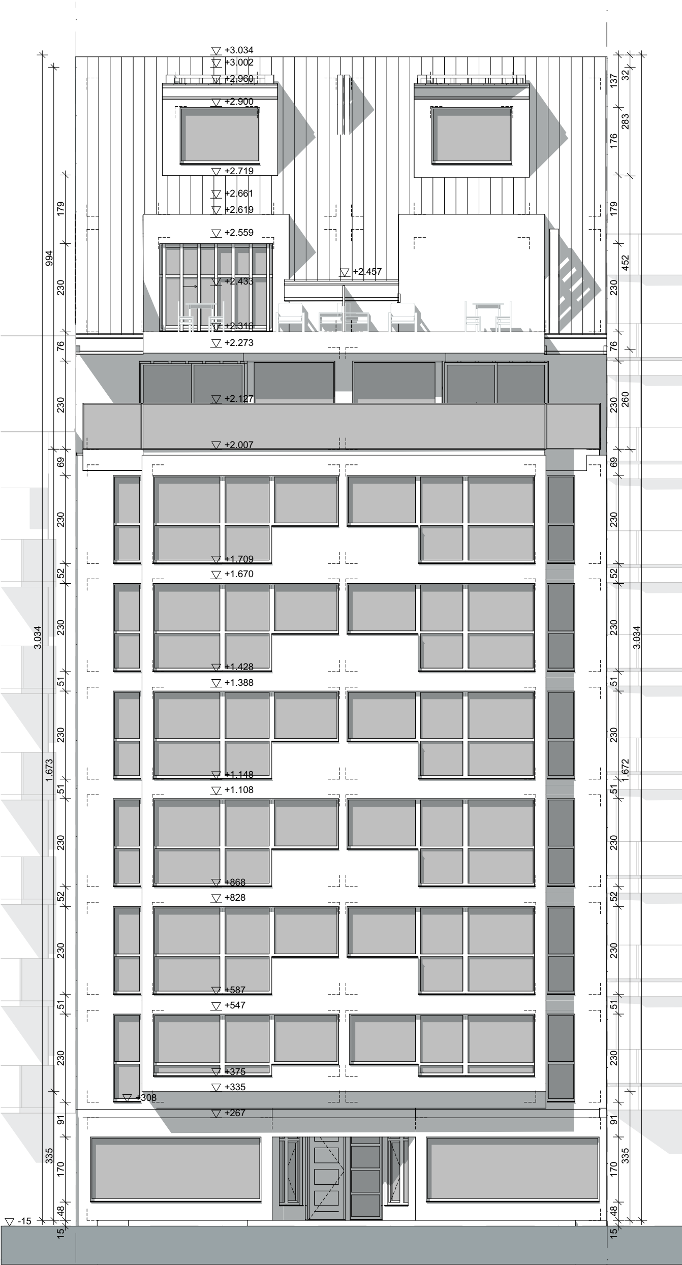
G1 Voorgevel (Zeedijk-Heist) 1:100
