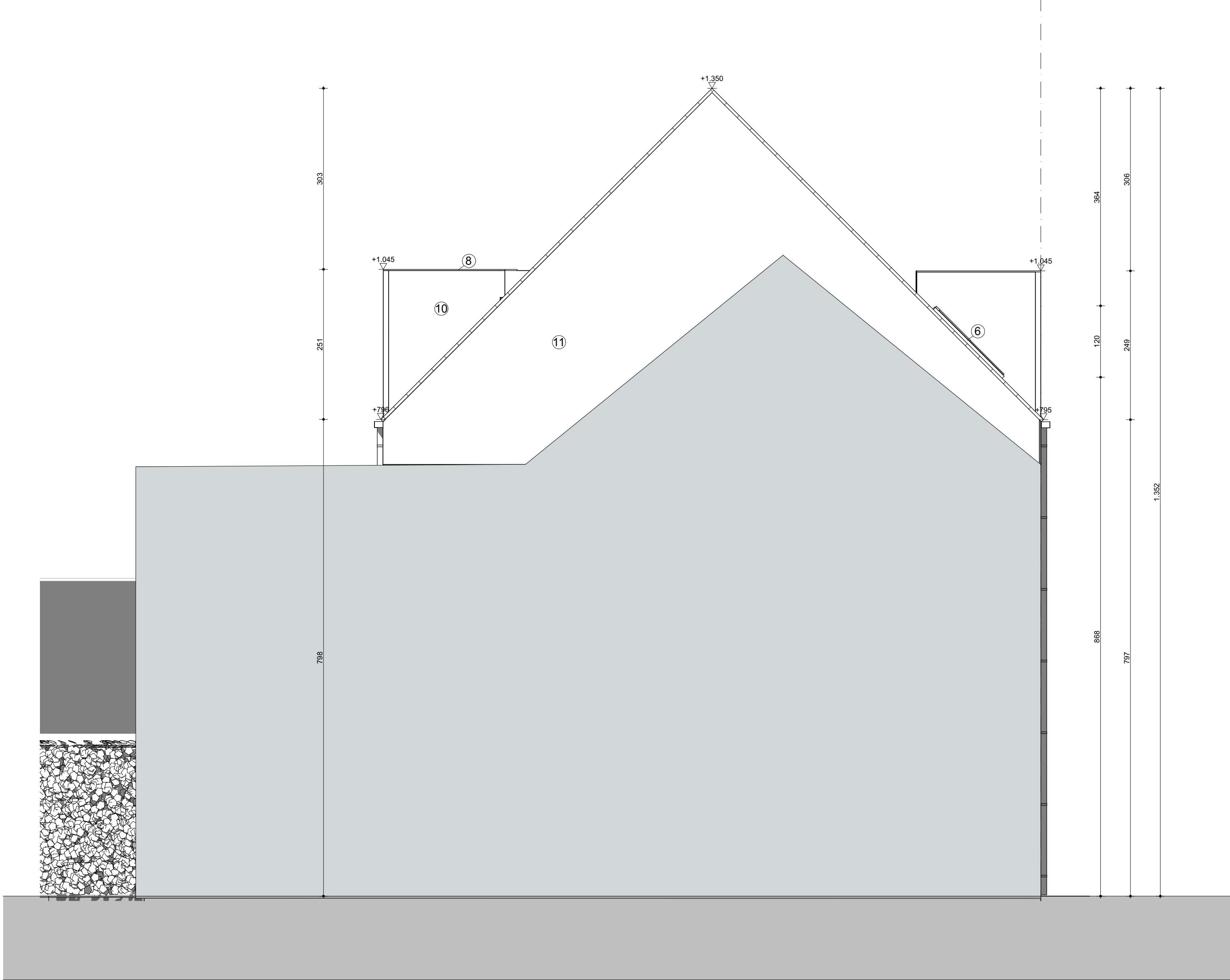
G4 Linkergevel 1:50
