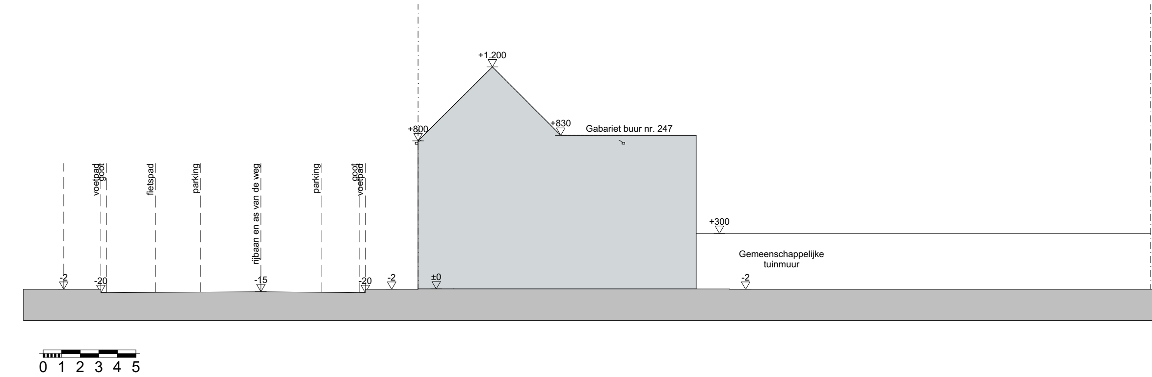
1.1 terreinprofiel BT 1:200
