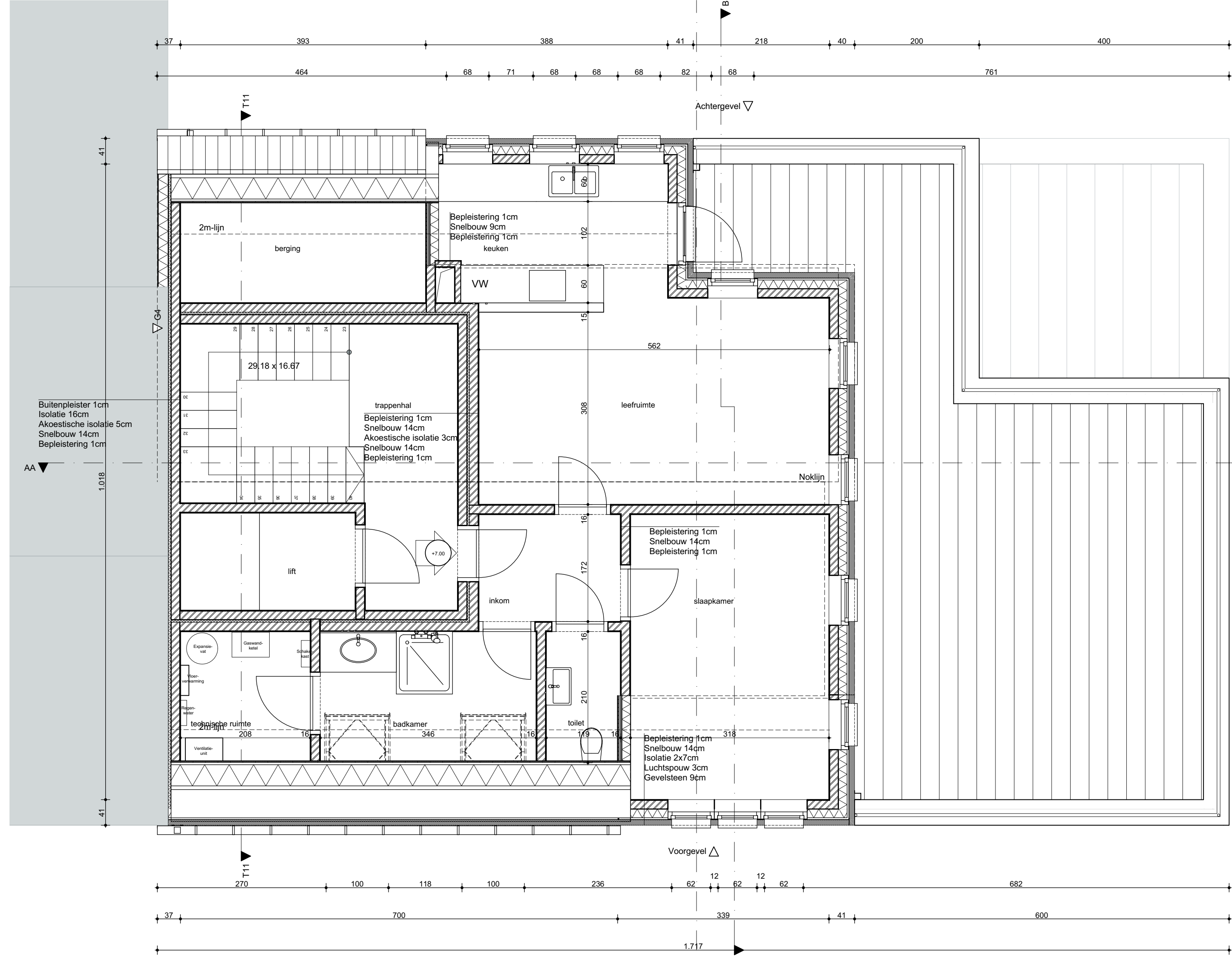
2. 2e verdieping 1:50
