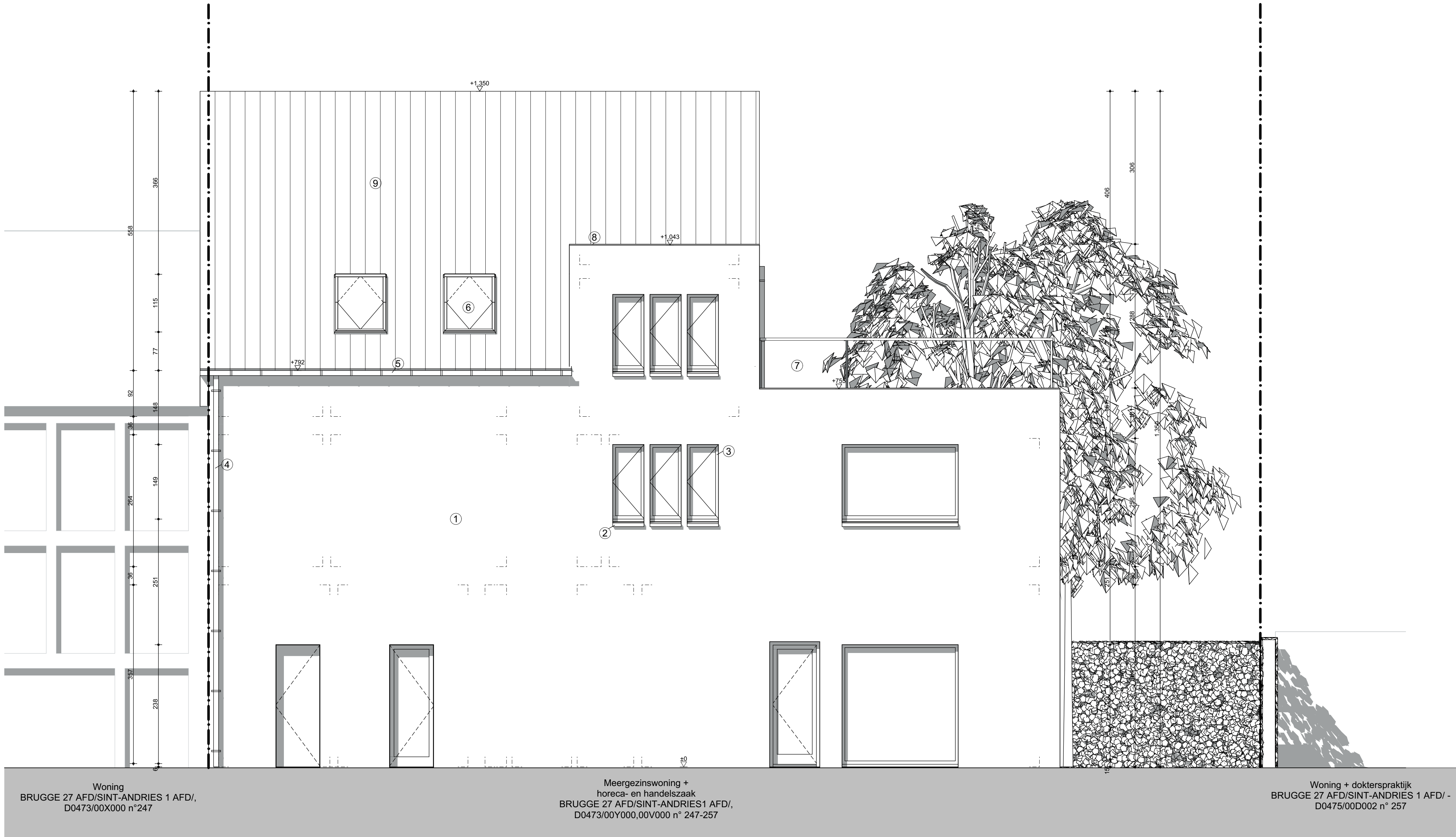
G1 Voorgevel 1:50
