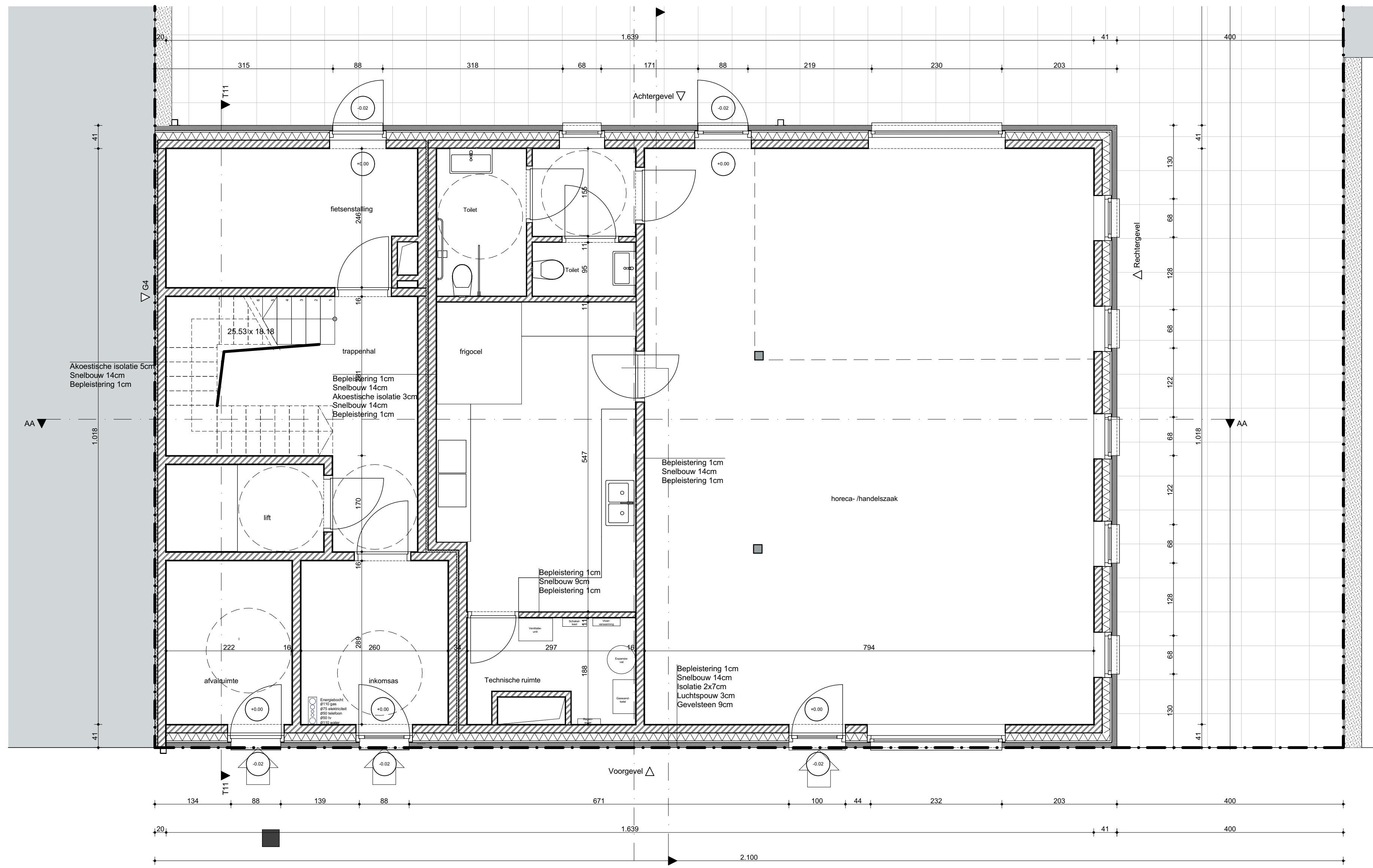
0. Gelijkvloers 1:50
