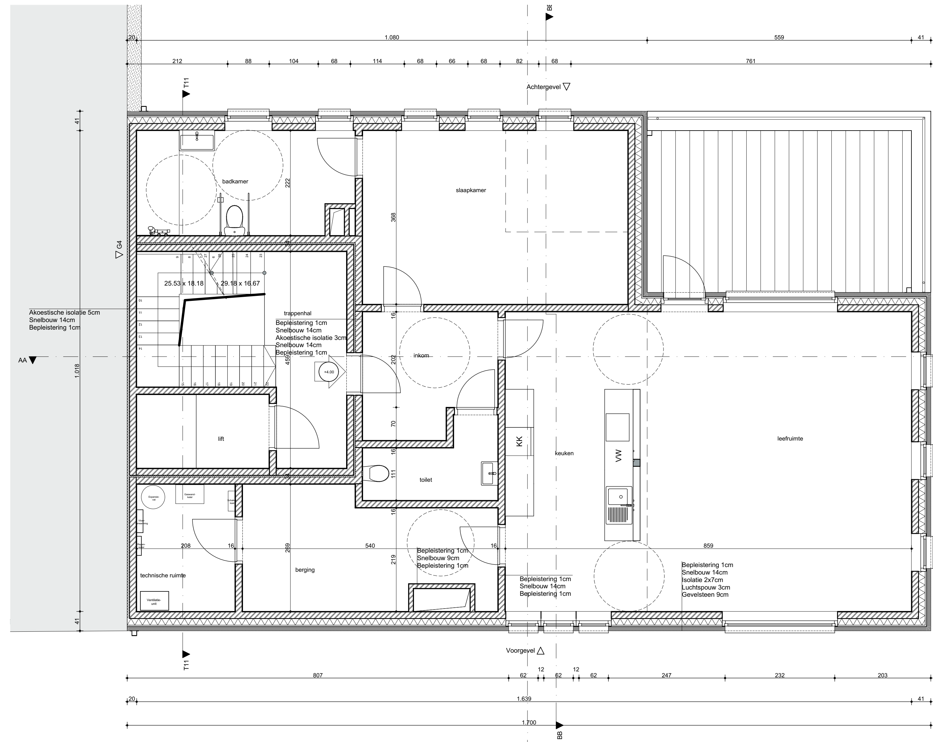
1. 1e verdieping 1:50
