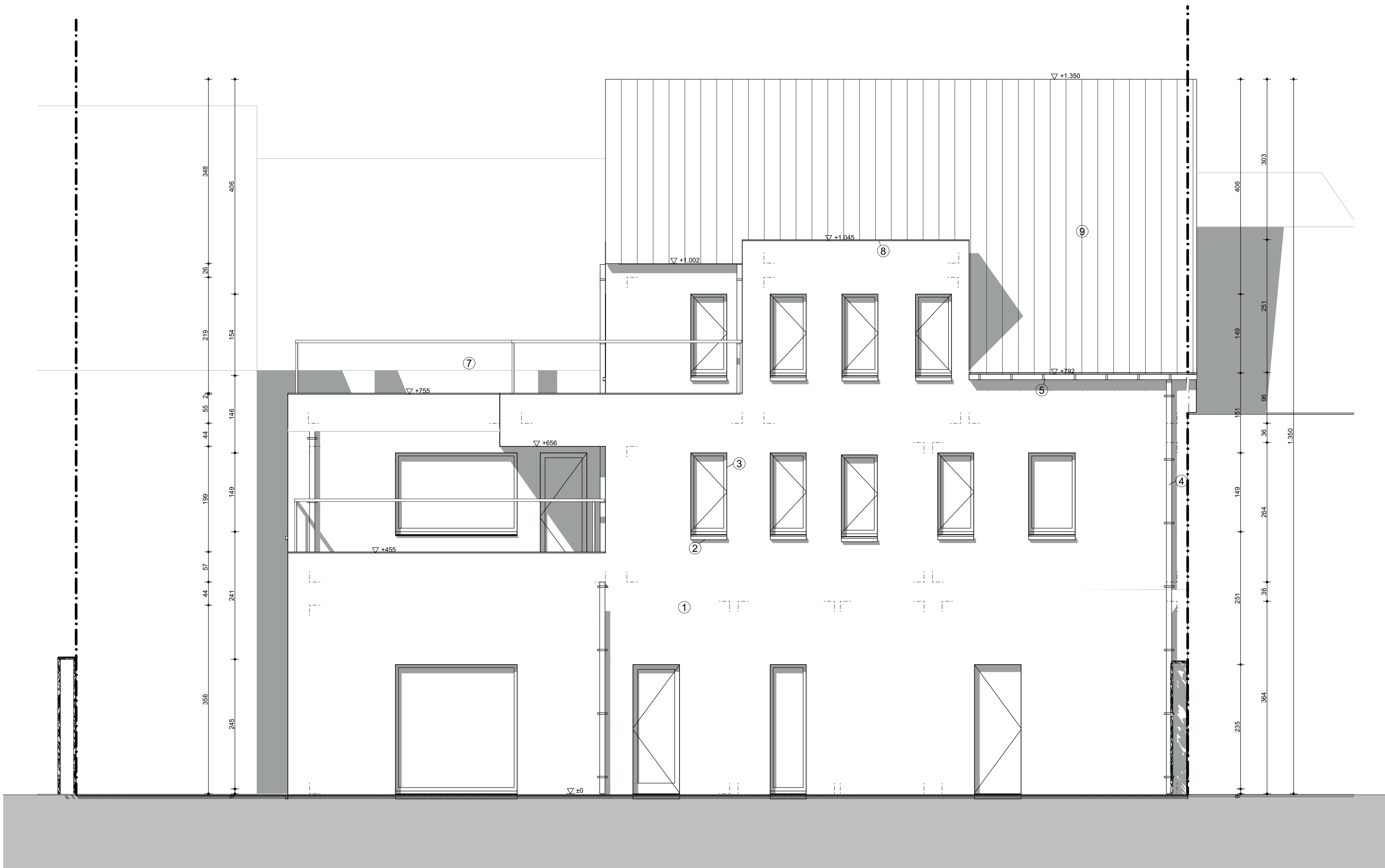
G3 Achtergevel 1:50
