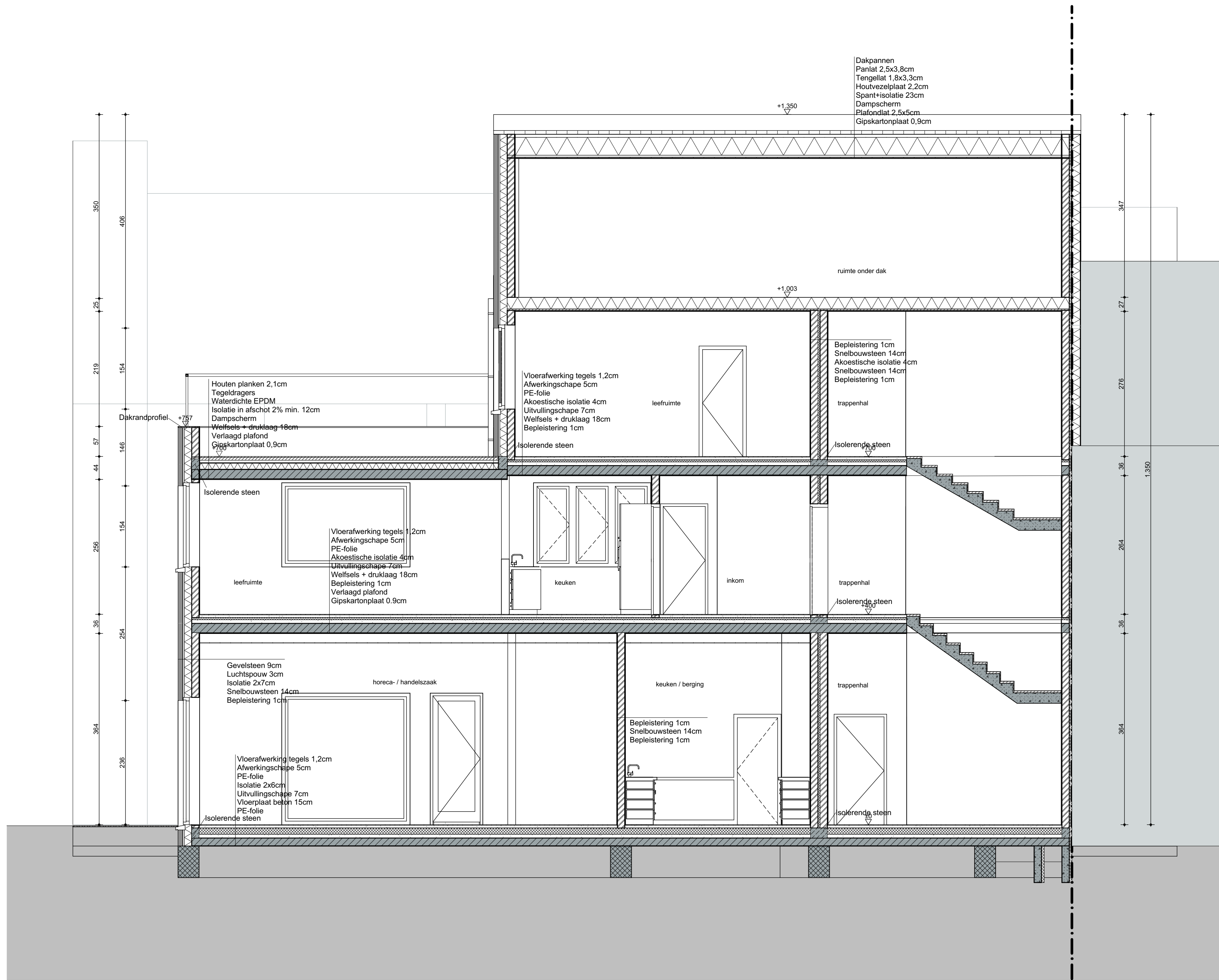
AA snede aa 1:50
