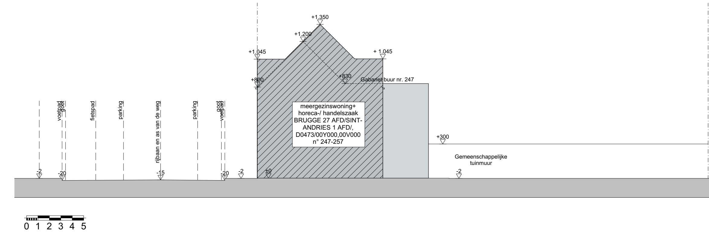
1.2 terreinprofiel NT 1:200
