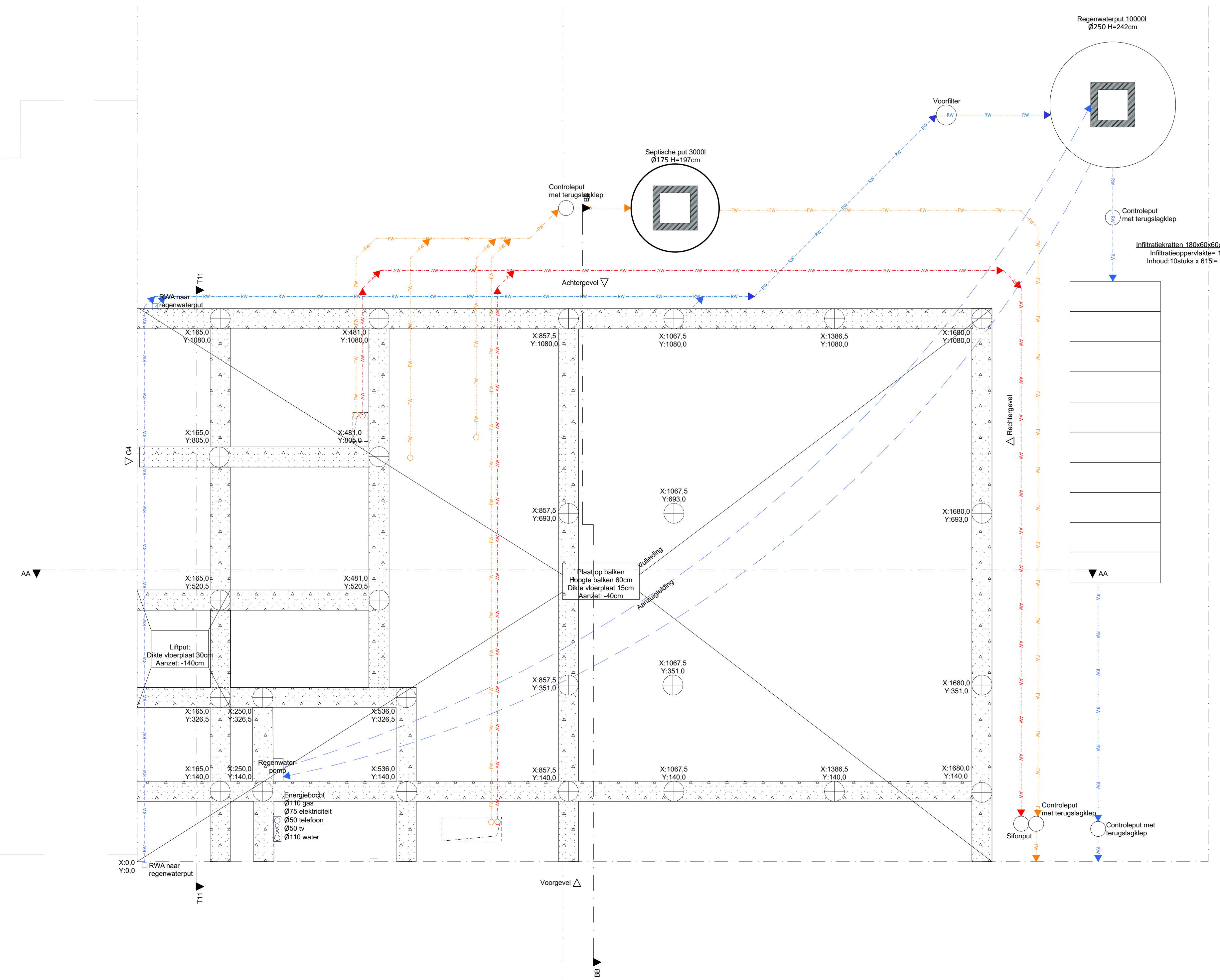
0. Gelijkvloers 1:50
