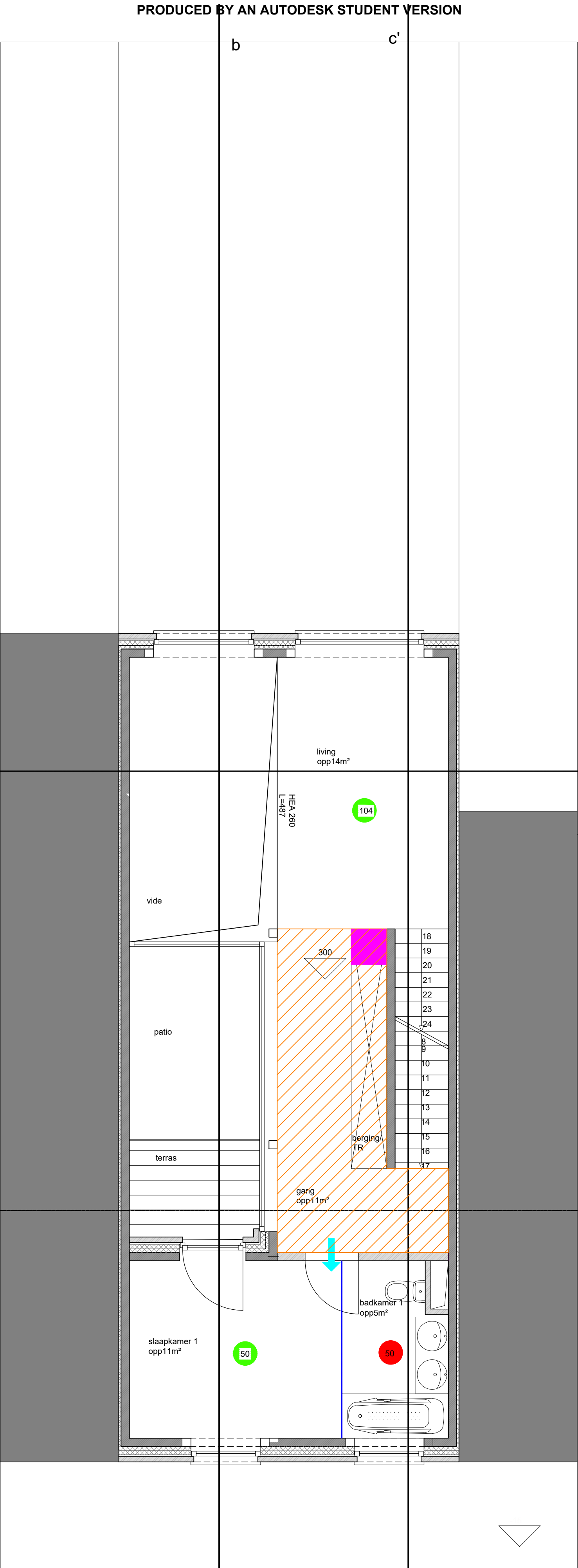
eerste verdiep 1/50
