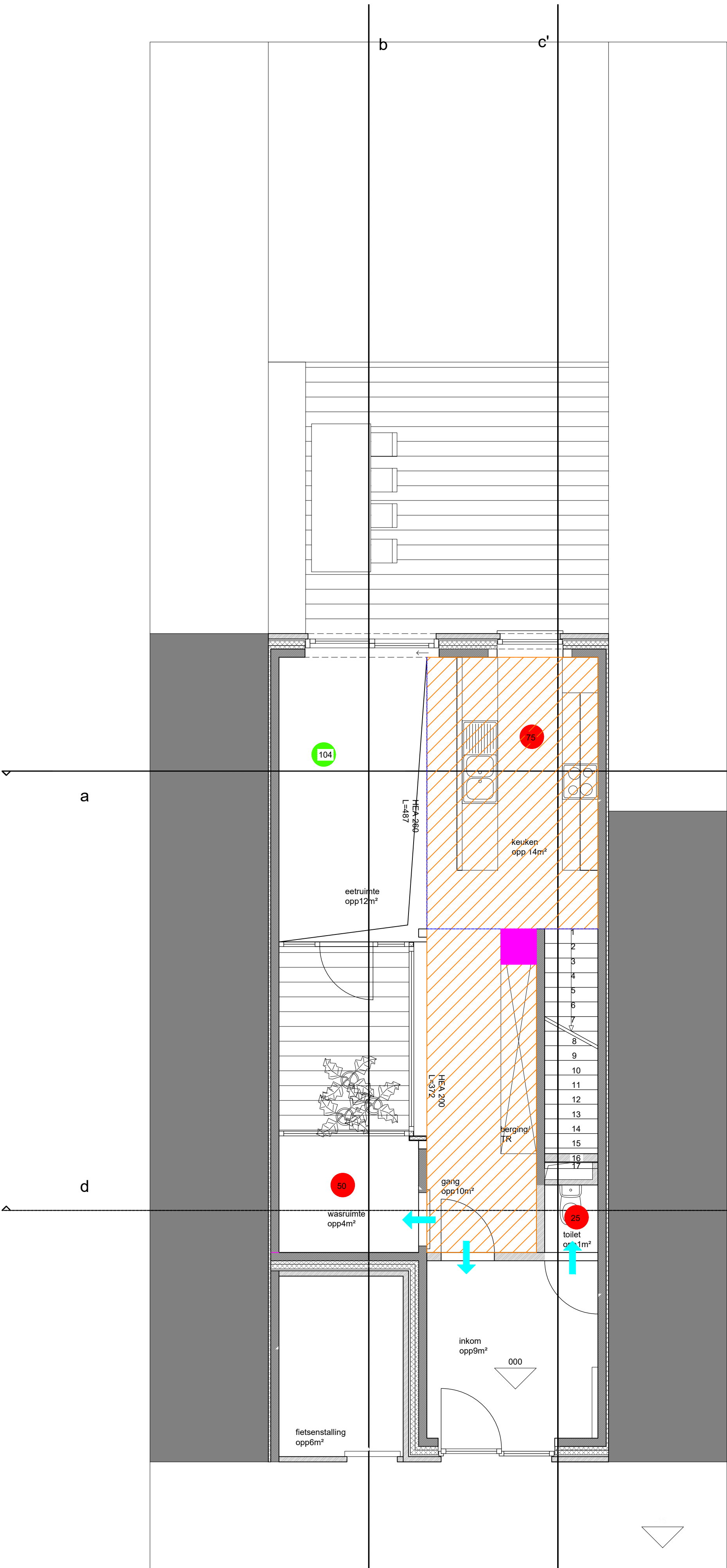
grondplan 1/50
